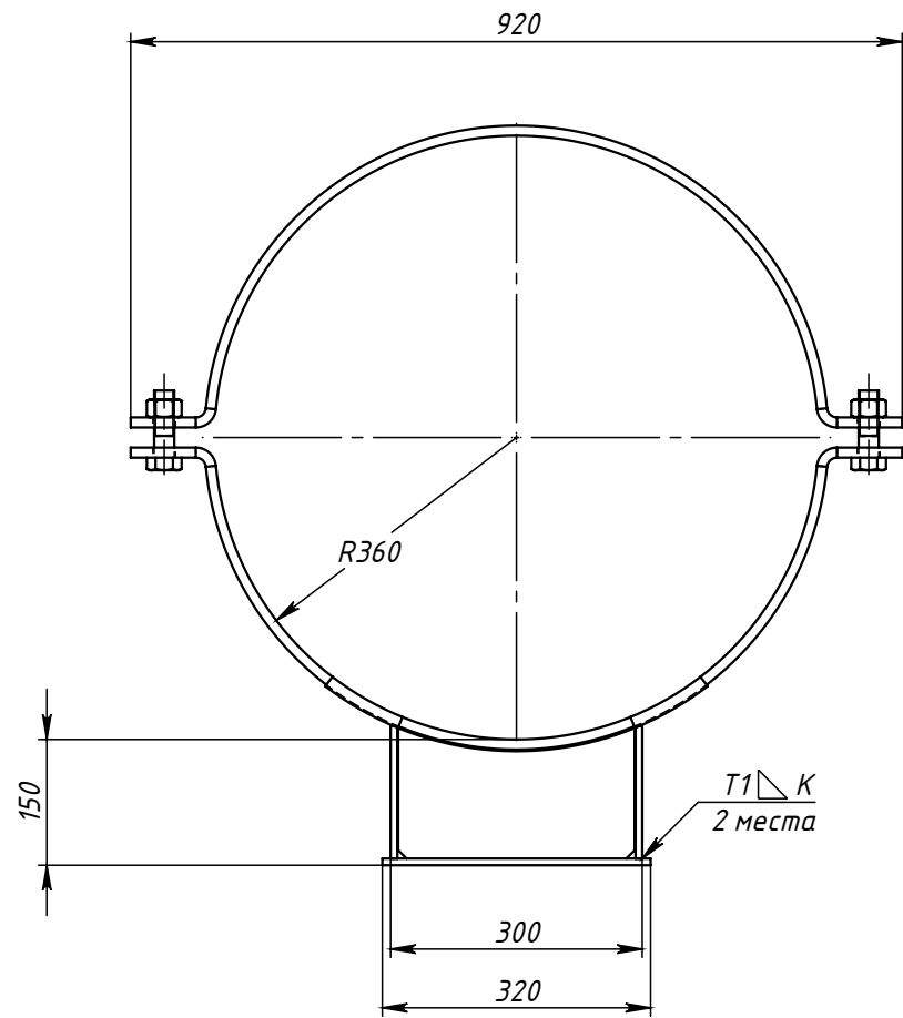
Поз.3 (Хомут)
