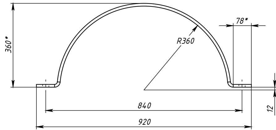
Поз.3 (Хомут) развертка
